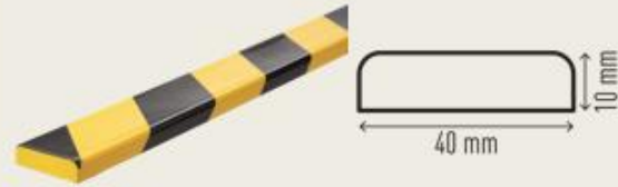
Profil S10
