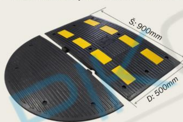
LP900 - Modularna jedinica 50cm x 90cm x 4,5cm
