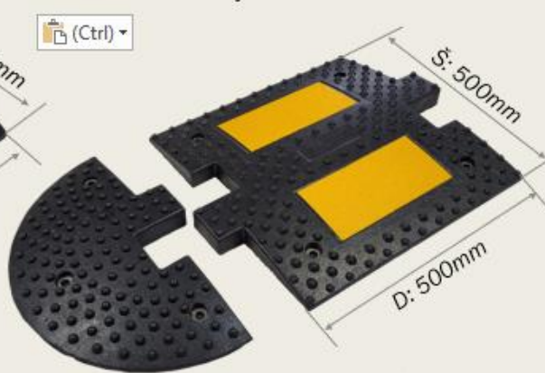
LP500 - Modularna jedinica 50cm x 50cm x 5cm
